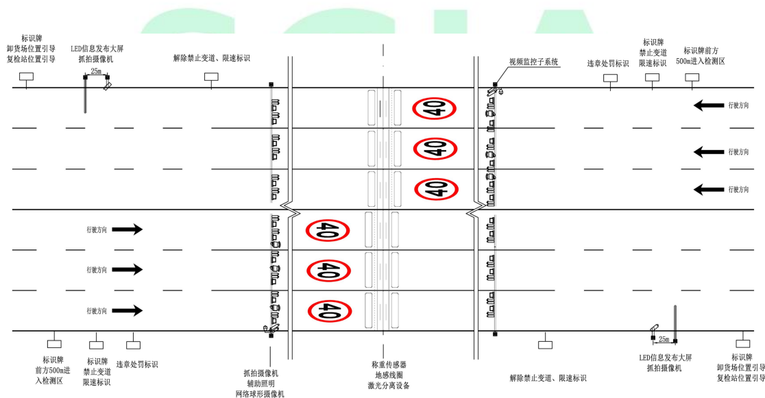
图3 不停车检测系统设备安装布置示意图
